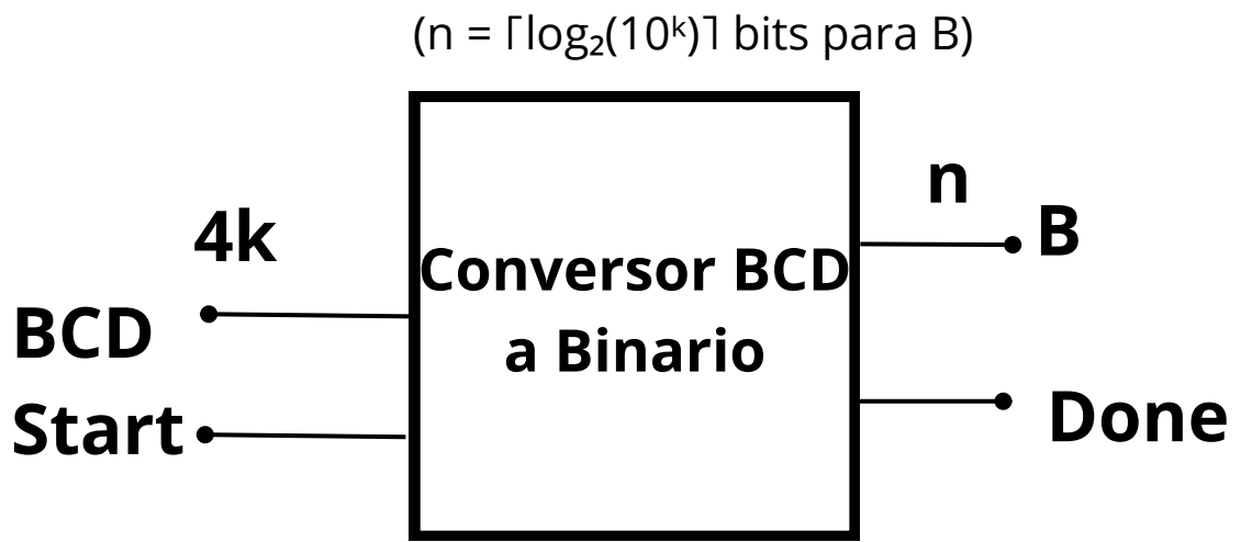
Diagrama de caja negra Reverse Double Dabble
